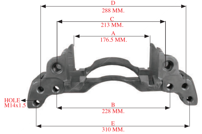
290K102 > BALATA TAŞIYICI - R - 17.5" CARRIER - R - 17.5"
