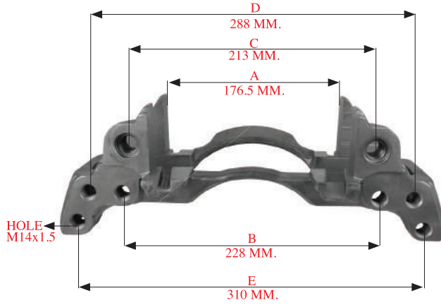
290K101 > BALATA TAŞIYICI - L - 17.5" CARRIER - L - 17.5"
